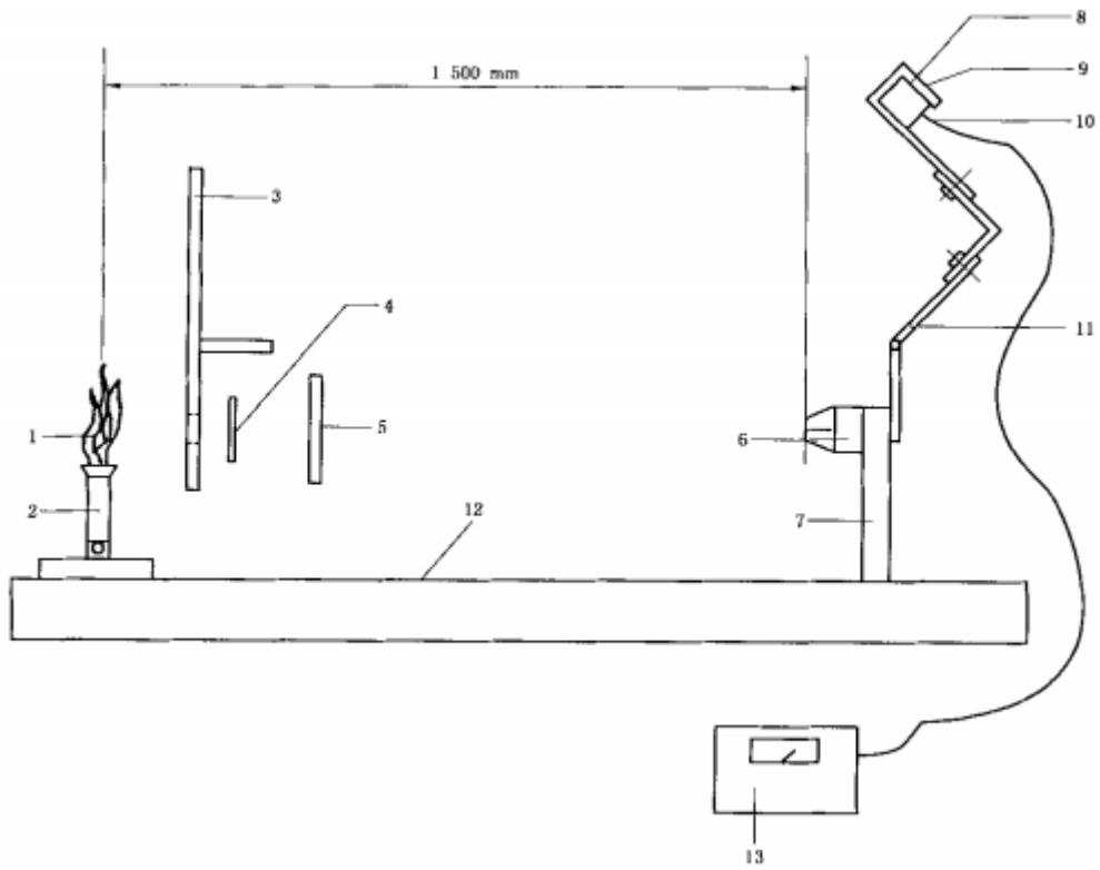
图 1 红外火焰试样检测装置结构图
