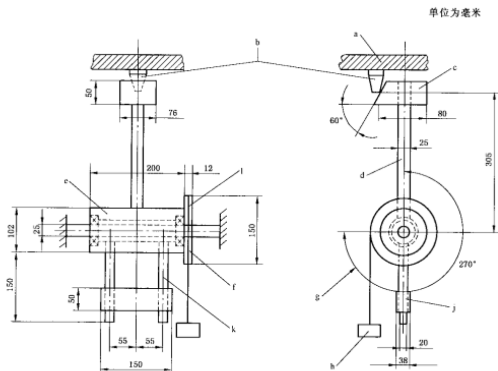
图 6 碰撞试验装置结构图
