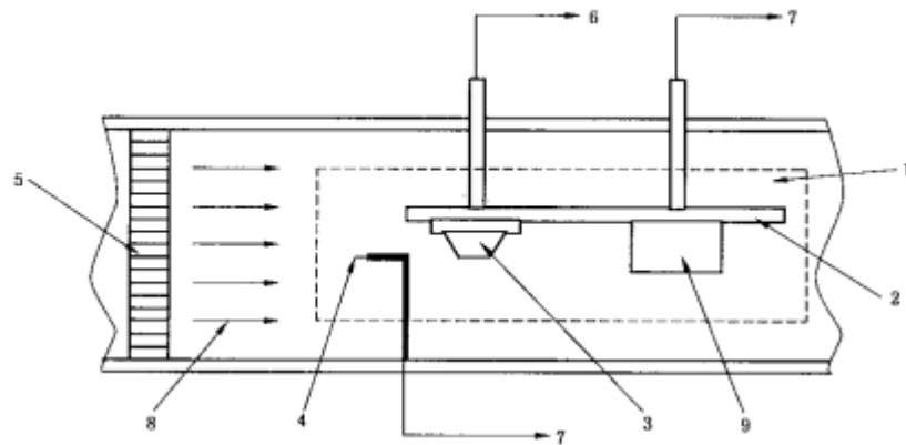
图 A.1 探测器、试验仪器布置图
