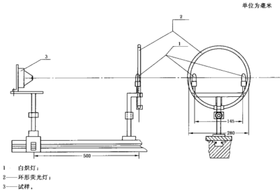
图3 环境光线干扰模拟装置结构图
